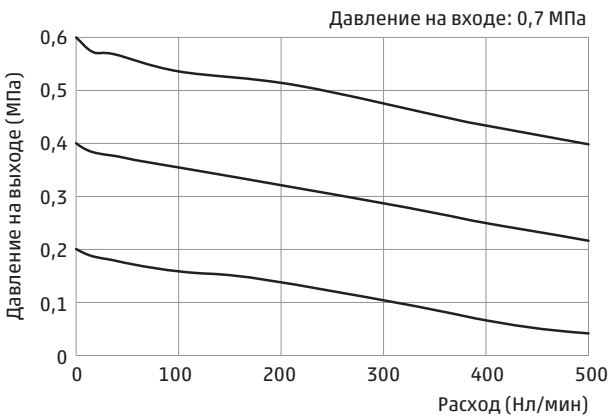
Расходная характеристика серии СС300 / СС305
