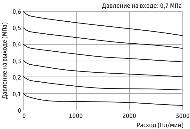
Расходная характеристика серии СС310 / СС315
