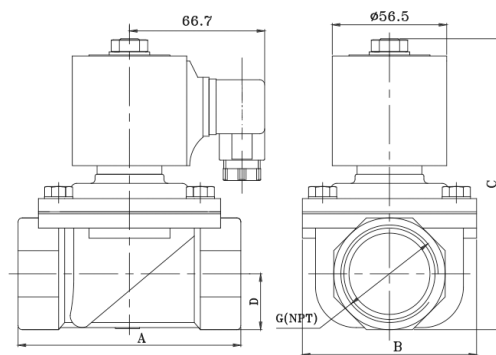
DN40 – DN50 (катушка S71B)
