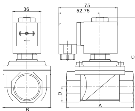
DN15 – DN32 (катушка S91B)
