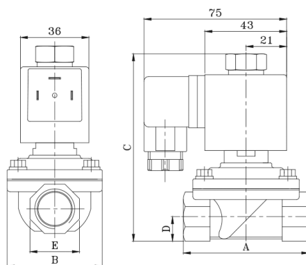
DN12 – DN25 (катушка S91BT)
