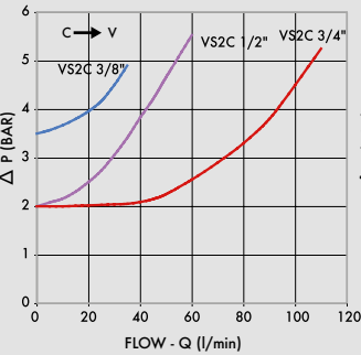
PERDITE DI CARICO PRESSURE DROP CURVE
