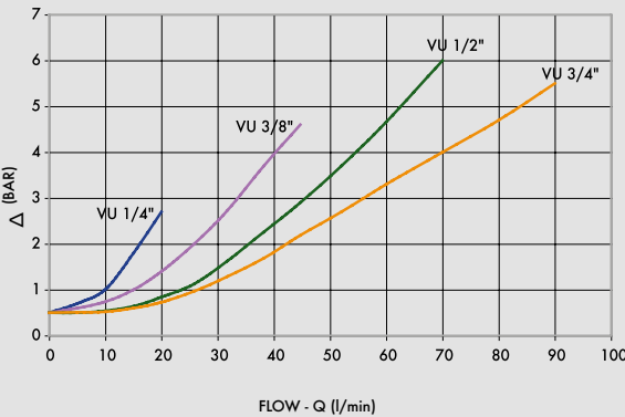
PERDITE DI CARICO PRESSURE DROP CURVE
